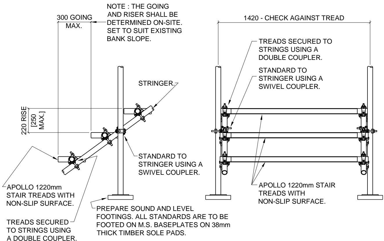
ELEVATION
